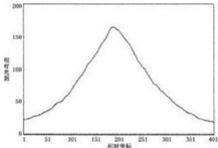
图 5 平滑处理后相对光强曲线
